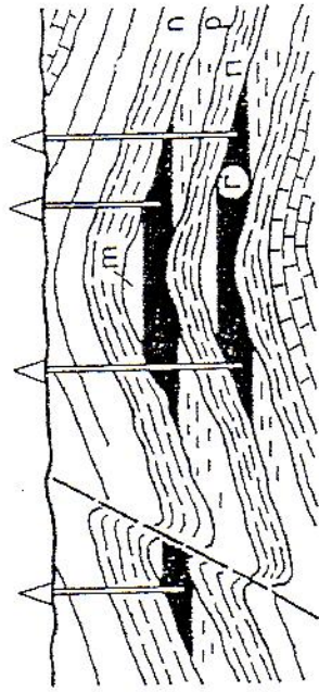
Obr. 61. Schéma nařazeného ložiska v antiklinálním ohybu vrstev n — nepropustné vrstvy; p — propustné vrstvy; f — ropa; m — proplyněné vrstvy
