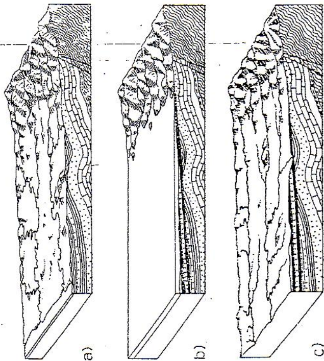
Obr. 47. Příklad transgrese a regrese moře (podle C. B. Browna a F. Debenhamů)
