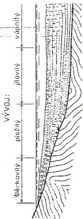
Obr. 46. Vývoj sedimentu, příklad facielní změny sedimentace
