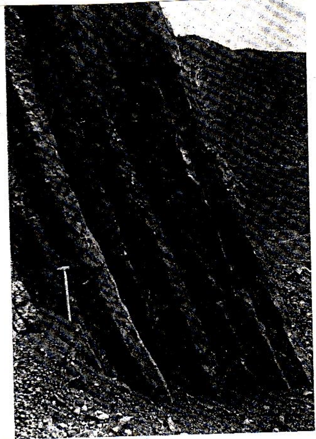
Obr. 35. Sloupcovitá odlučnost čediče (foto B. Červený)
