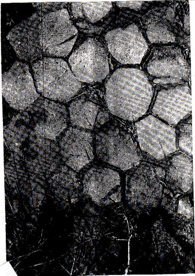
Obr. 34. Sloupcovitá odlučnost čediče; pohled na hlavy čedičových sloupců. Kamenický Šenov (foto J. Vachtl)
