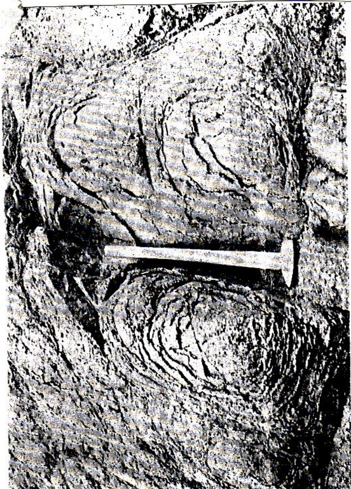
Obr. 33. Koncentrický kulovitý rozpad diábasu Loděnice u Berouna (foto Q. Záruba)
